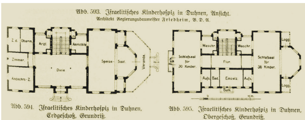
Grundriss des israelitischen Kinder-Hospiz in Duhnen
