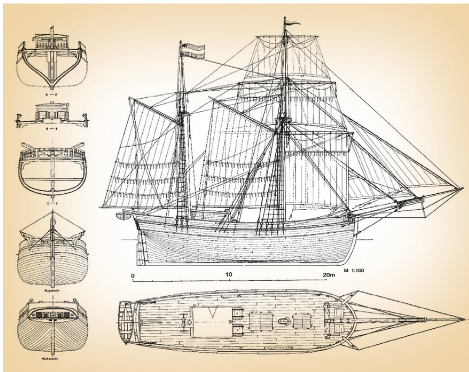
Abbildung des Plans der Brigg HELENE aus dem Jahr 1828
